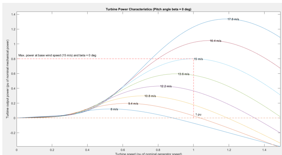
Рисунок 2 – Потужність турбіни у відносних одиницях( \beta=0 ) при відповідних значеннях швидкості вітру
