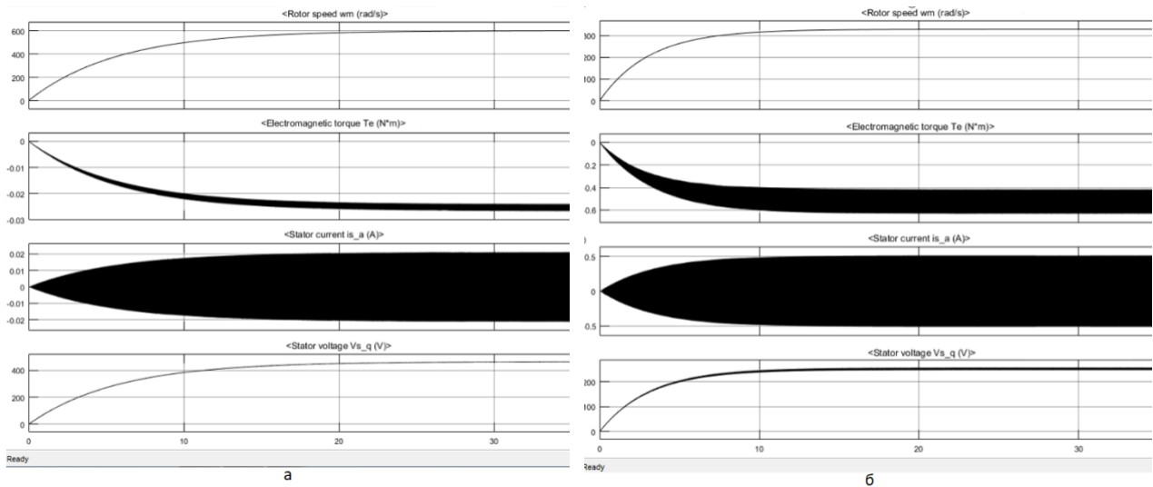
Рисунок 3 – Параметри генератора:
