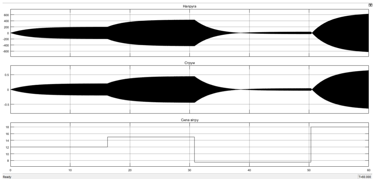
Рисунок 5 – Залежність вихідної напруги та струму від швидкості вітру (при \beta=0 )
